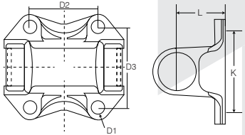
FLANGE YOKES
