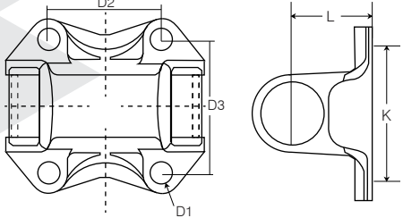
FLANGE YOKES
